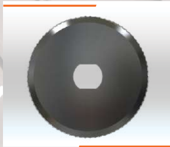
DISCO SERRILHADO FIO ÚNICO Ø125x25-30x2mm Cód. IMESC: 824201 Ref. Original: [REDACTED]
