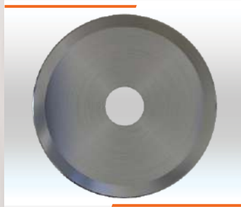
DISCO FIO DUPLO Ø150x32x2mm Cód. IMESC: 86128 Ref. Original: [REDACTED]
