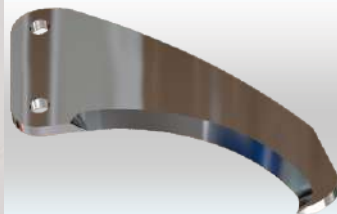
LÂMINA TESOURA DA DESNUCA 307x330x12,60mm Cód. IMESC: 637577 Ref. Original: [REDACTED]
