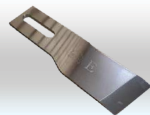
LÂMINA ESQUERDA FHF-XB 36x129x4mm Cód. IMESC: 446448 Ref. Original: [REDACTED]
