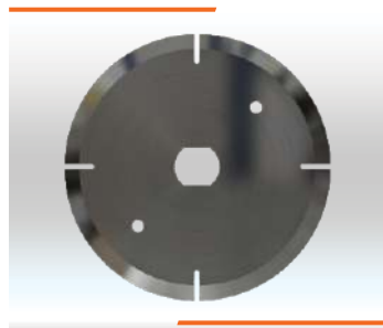
DISCO FIO ÚNICO Ø175x25-30x2mm 4T Cód. IMESC: 628988 Ref. Original: [REDACTED]
