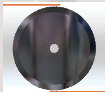
DISCO FIO DUPLO ONDULADO ZIG-ZAG Ø295x32x3mm Cód. IMESC: 112118 Ref. Original: [REDACTED]
