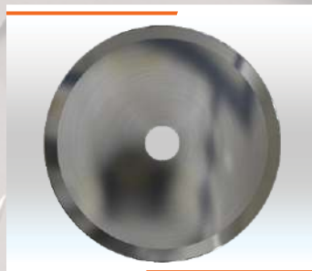
DISCO FIO DUPLO Ø270x40x3mm Cód. IMESC: 79992 Ref. Original: [REDACTED]
