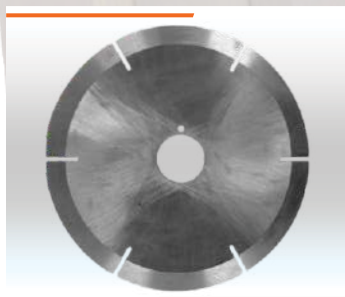
DISCO FIO ÚNICO Ø175x32x2mm 6T Cód. IMESC: 112041 Ref. Original: [REDACTED]
