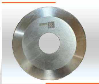
DISCO FIO DUPLO Ø110x32x2mm Cód. IMESC: 692250 Ref. Original: [REDACTED]
