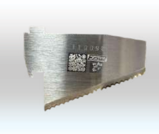
LÂMINA SERRILHADA FIO DUPLO 61x41x1,50mm Cód. IMESC: 250644 Ref. Original: [REDACTED]
