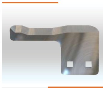
LÂMINA DIREITA CORTE DO LOMBO 96X54X6MM Cód. IMESC: 243347 Ref. Original: [REDACTED]
