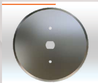
DISCO SERRILHADO FIO ÚNICO Ø250X(25-30)X2MM
