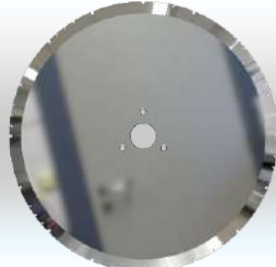
DISCO DE CORTE D260x25x5mm Esquerdo Cód. IMESC: 112076 Ref. Original: [REDACTED]
