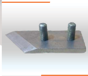
LÂMINA ESQUERDA 25x70x4mm Cód. IMESC: 894670 Ref. Original: [REDACTED]
