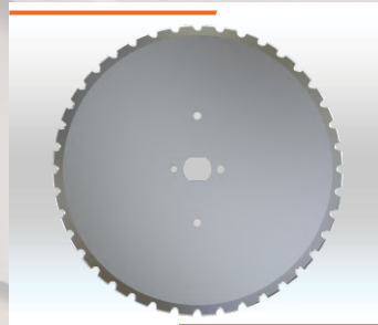
DISCO FIO DUPLO Ø300x25-30x3mm 40T Cód. IMESC: 793015 Ref. Original: 673314
