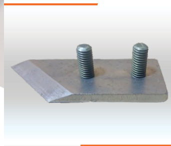
LÂMINA ESQUERDA 25x70x4mm Cód. IMESC: 894670 Ref. Original: 176555
