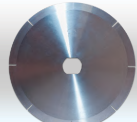
DISCO SANGRADOR SEMIL Ø200x25-30x2mm 8T
