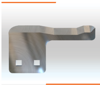
LÂMINA ESQUERDA CORTE DO LOMBO 96X54X6MM Cód. IMESC: 931956 Ref. Original: 3982547B
