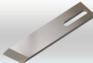
LÂMINA DIREITA 30x133,50x4mm Cód. IMESC: 112122 Ref. Original: 4430032A
