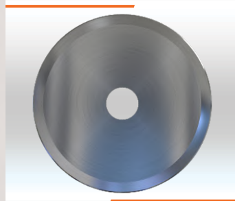
DISCO FIO DUPLO Ø175x32x2mm Cód. IMESC: 693948 Ref. Original: 91 200 1753
