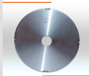
DISCO FIO ÚNICO Ø200x32x2,50mm 4T Cód. IMESC: 498341 Ref. Original: 625954
