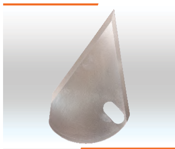
LÂMINA GOTA 98x155x3mm Cód. IMESC: 424301 Ref. Original: 616347
