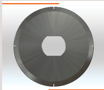
DISCO FIO DUPLO Ø100x25-30x2mm 4T Cód. IMESC: 112009 Ref. Original: 629326
