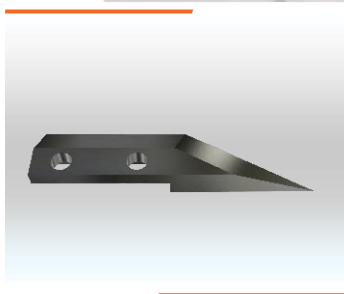
LÂMINA DIREITA FIO ÚNICO 25x95x10mm Cód. IMESC: 606465 Ref. Original: 901556
