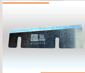
LÂMINA DIREITA JLR 90X31X2,5MM Cód. IMESC: 771622 Ref. Original: 617359A
