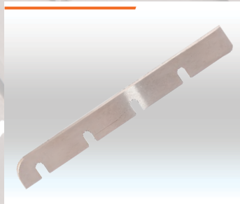
LÂMINA 25x220x1,20mm Cód. IMESC: 469837 Ref. Original: 256438
