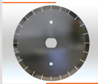
DISCO FIO ÚNICO Ø200X(25-30)X2MM 24T Cód. IMESC: 771032 Ref. Original: 3923256
