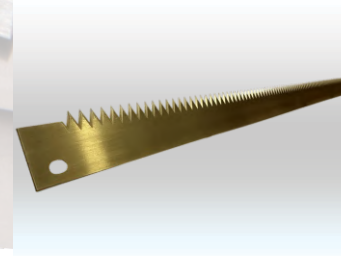
LÂMINA PARA SELADORA PACMAC 27,50x515x1,5MM
