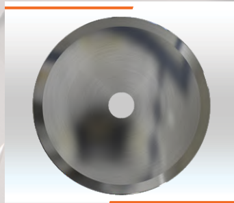
DISCO FIO DUPLO Ø270x40x3mm Cód. IMESC: 79992 Ref. Original: 08.24.000.003
