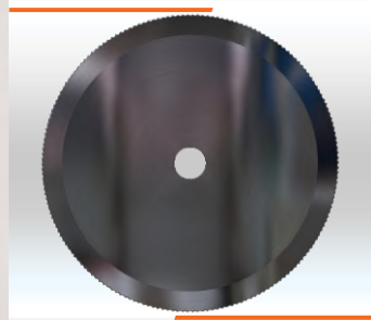
DISCO FIO DUPLO ONDULADO ZIG-ZAG Ø295x32x3mm Cód. IMESC: 112118 Ref. Original: 174250
