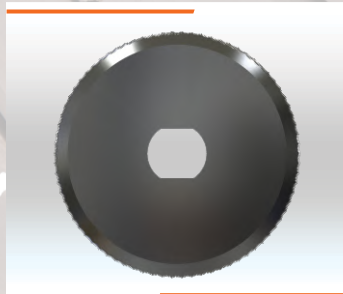
DISCO SERRILHADO FIO ÚNICO Ø125x25-30x2mm Cód. IMESC: 824201 Ref. Original: 3960622
