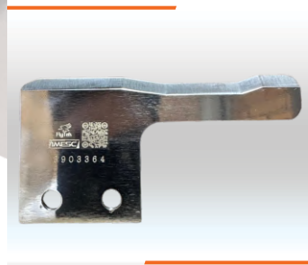
LÂMINA ESQUERDA FHF-XB 96X50X4MM Cód. IMESC: 736866 Ref. Original: 3903364
