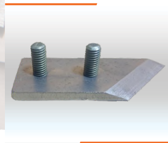
LÂMINA DIREITA 25x70x4mm Cód. IMESC: 610473 Ref. Original: 176556
