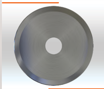
DISCO FIO DUPLO Ø150x32x2mm Cód. IMESC: 86128 Ref. Original: 0062583
