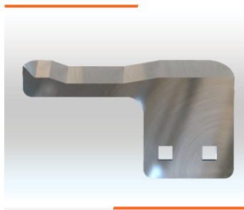
LÂMINA DIREITA CORTE DO LOMBO 96X54X6MM Cód. IMESC: 243347 Ref. Original: 3982546B
