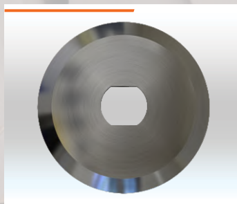
DISCO FIO ÚNICO Ø110x25-30x2mm Cód. IMESC: 86212 Ref. Original: 555710
