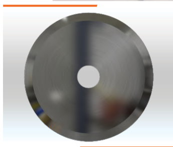
DISCO FIO ÚNICO Ø125x22x2mm Cód. IMESC: 112014 Ref. Original: 438394
