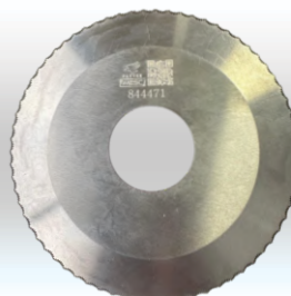
DISCO SERRILHADO LINGO Ø110x32x2mm
