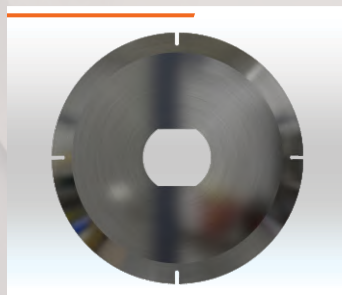
DISCO FIO ÚNICO Ø110x25-30x2mm 4T Cód. IMESC: 112012 Ref. Original: 629925
