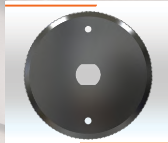
DISCO SERRILHADO FIO ÚNICO Ø150x25-30x2mm Cód. IMESC: 163054 Ref. Original: 3994454
