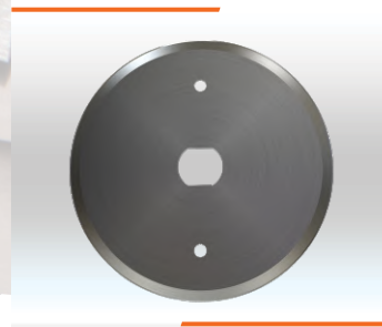
DISCO FIO ÚNICO Ø175x25-30x2mm Cód. IMESC: 748343 Ref. Original: 507971
