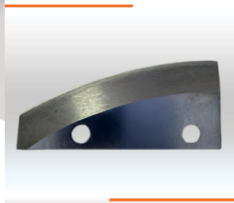
LÂMINA CORTE DA COXA ESQUERDA 65X30X2,50MM Cód. IMESC: 166557 Ref. Original: 0990.IDC1.004.00
