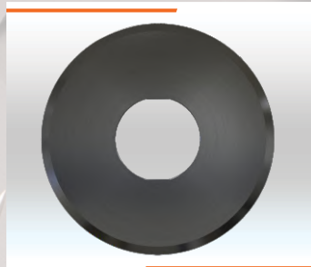
DISCO FIO ÚNICO Ø150x52,5-55x2mm Cód. IMESC: 112016 Ref. Original: 4486805
