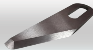
LÂMINA FIO DUPLO 30x114x4mm Cód. IMESC: 112068 Ref. Original: 3955523
