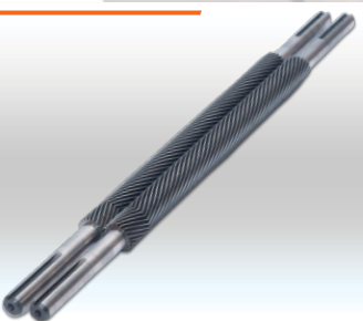
ROLETE DE MOELA SEMIL COM INVERSÃO Ø26x495mm
