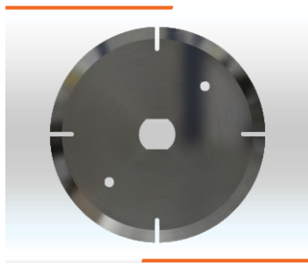
DISCO FIO ÚNICO Ø175x25-30x2mm 4T Cód. IMESC: 628988 Ref. Original: 518391
