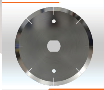
DISCO FIO ÚNICO Ø175x25-30x2mm 8T Cód. IMESC: 112020 Ref. Original: 622400
