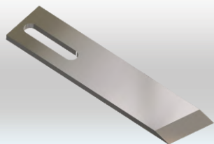
LÂMINA ESQUERDA 30x133,50x4mm Cód. IMESC: 112120 Ref. Original: 4430031A
