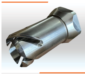
NAVALHA TUBULAR 4T ESQUERDA Cód. IMESC: 259906 Ref. Original: 302838641
